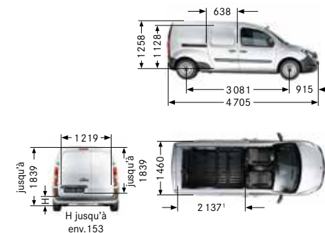
Fourgon en version extra longue avec empattement de 3 081 mm
