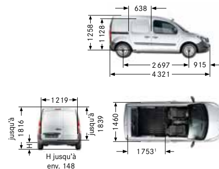
Fourgon version longue, empattement de 2 697 mm
