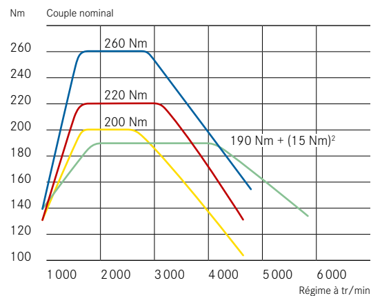
Courbes de couple
