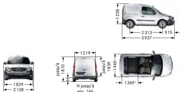
Fourgon version courte, empattement de 2 313 mm
