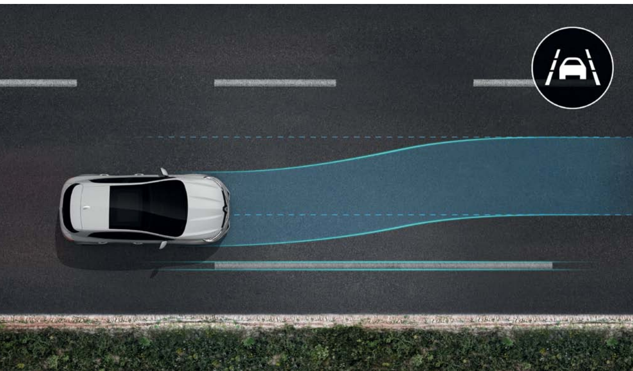
système d’aide au maintien dans la voie Il applique une correction sur le volant pour ramener le véhicule dans sa voie si vous n’enclenchez pas votre clignotant.
