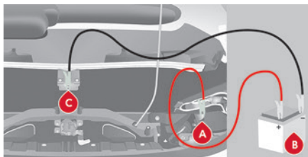
A. Point métallique positif de votre véhicule B. Batterie de secours
