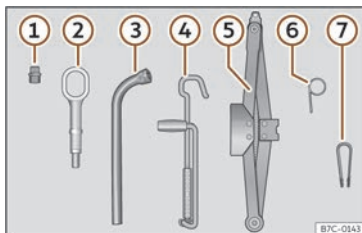
Fig. 34 Dans le coffre à bagages, sous le revêtement du plancher de chargement : outillage de bord.
