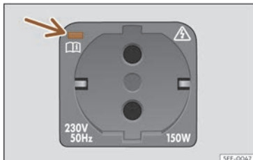
Fig. 130 Du côté droit du coffre à bagages : prise de courant de 230 volts.
