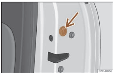
Fig. 81 Verrouillage d'urgence de la porte.
