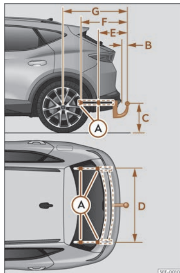
Fig. 193 Cotes et points de fixation pour l'installation d'un dispositif d'attelage en deuxième monte.
