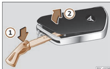
Fig. 74 Clé du véhicule : ouvrir le cache du compartiment de la pile.
