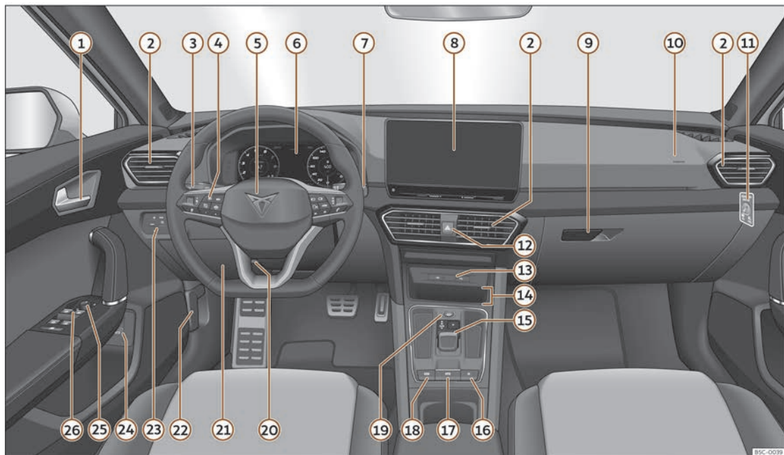
Fig. 51 Poste de conduite.
