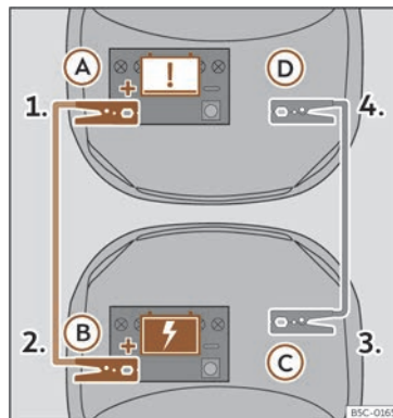
Fig. 43 Schéma de branchement pour les véhicules équipés du système Start-Stop.
