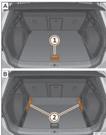
Fig. 117 Plancher de coffre à bagages modulable : A position haute ; B position basse.
