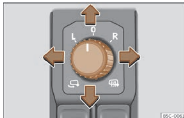
Fig. 100 Détail de la porte du conducteur : commande du rétroviseur extérieur.
