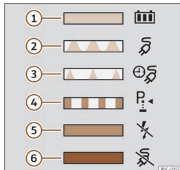
Fig. 200 Sur la face intérieure de la trappe de la prise de charge de la batterie : autocollant avec informations sur l'indicateur de l'opération de charge.
