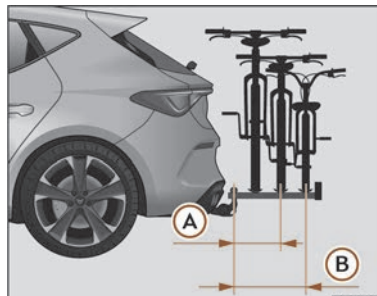
Fig. 197 Schéma de représentation de l'encorbellement maximal de la charge sur un porte-vélo pour deux ou trois vélos.
