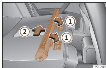
Fig. 183 Monter le filet de séparation sur le dossier de la banquette arrière.
