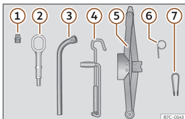
Fig. 203 Dans le coffre à bagages, sous le plancher de la surface de chargement : outillage de bord.
