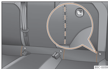
Fig. 41 Sièges arrière : fentes découpées pour accéder aux anneaux de fixation ISOFIX/i-Size.
