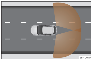
Fig. 125 Zones de détection des capteurs.
