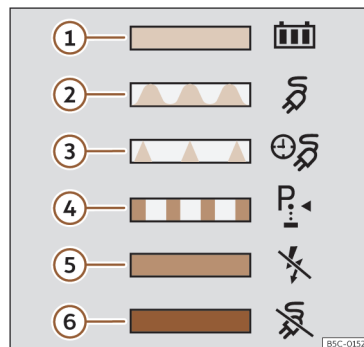
Fig. 58 Sur le côté intérieur de la trappe de la prise de charge de la batterie : autocollant avec information relative à l'indicateur de progression du rechargement.
