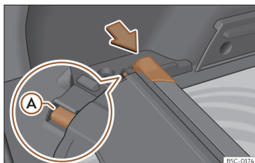
Fig. 178 Dans le coffre à bagages : logement pour ranger la plage enroulable.
