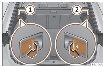
Fig. 98 Dans le coffre à bagages : leviers de déverrouillage du dossier arrière.
