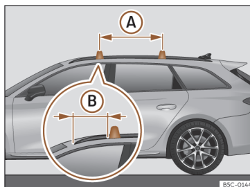
Fig. 192 Points de fixation des barres longitudinales pour la galerie porte-bagages du toit (Leon Sportstourer).
