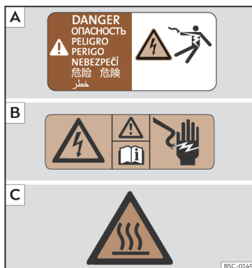
Fig. 52 Étiquettes d'avertissement.
