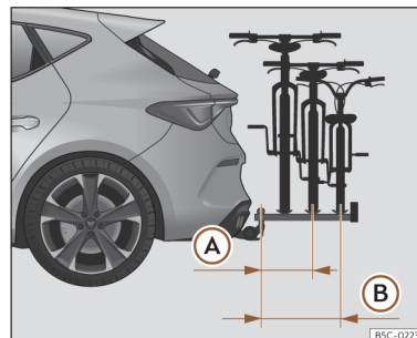
Fig. 197 Schéma de représentation de l'encorbellement maximal de la charge sur un porte-vélo pour deux ou trois vélos.
