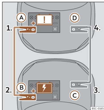
Fig. 206 Schéma de branchement pour les véhicules équipés du système Start-Stop.
