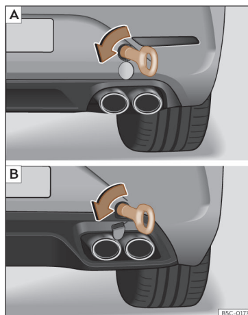
Fig. 210 Du côté droit du pare-chocs arrière : œillet de remorquage vissé. [A] Leon Sportstourer ; [B] Leon.
