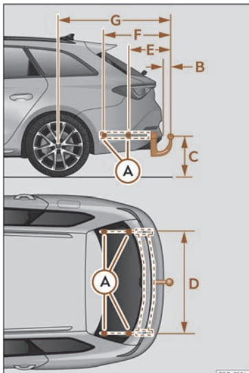
Fig. 206 Cotes et points de fixation pour le montage ultérieur d'un dispositif de remorquage.
