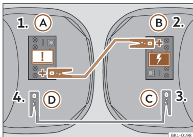
Fig. 185 Schéma de branchement des câbles de démarrage.
