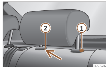
Fig. 88 Appui-tête arrière : démontage.
