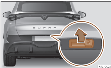
Fig. 77 Hayon arrière : ouverture de l'extérieur.
