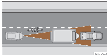
Fig. 122 Motocycliste circulant à l'avant hors du rayon d'action du capteur radar.
