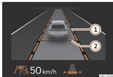
Fig. 129 Sur l'écran du combiné d'instruments : visualisation avec le régulateur actif (représentation schématique).
