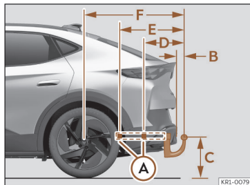
Fig. 179 Dispositif de remorquage : cotes et points de fixation.
