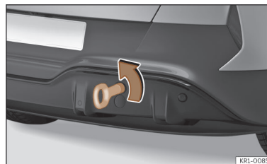
Fig. 189 Du côté droit du pare-chocs arrière : œillet de remorquage vissé.
