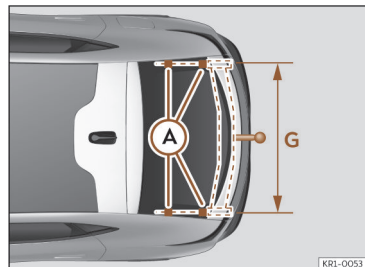
Fig. 180 Dispositif de remorquage : cotes et points de fixation.
