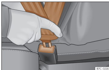
Fig. 21 Insérer la languette de la ceinture de sécurité dans son boîtier de verrouillage.
