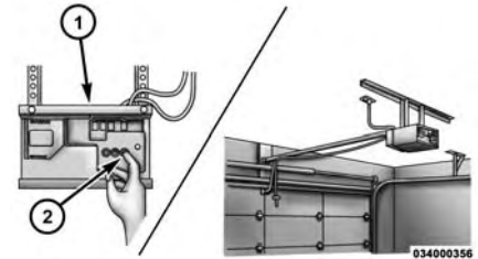
Programmation de l'ouvre-porte de garage
