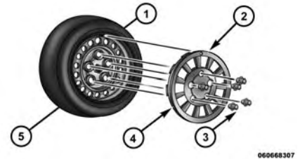
Pneu et enjoliveur de roue ou couvre-moyeu
