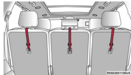
Montage de la courroie d'attache supérieure de la banquette de deuxième rangée (huit places)
