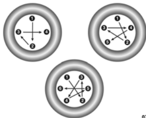
Modèles de couple de serrage
