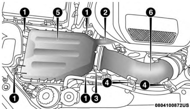
Couvercle du filtre à air du moteur et tube de prise d'air pur
