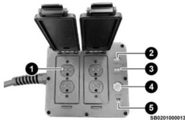
Boîtier d'alimentation
