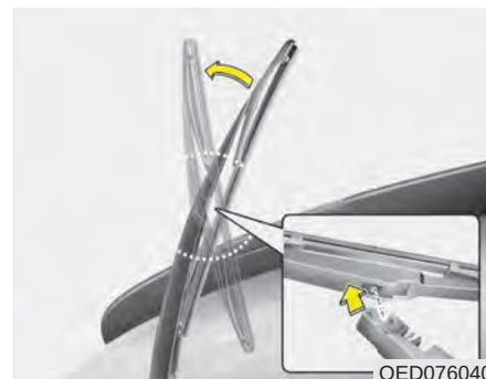
Lame d'essuie-glace de lunette
