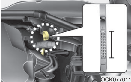
■ Moteur Lambda II 3,3L T-GDI (Essence)
