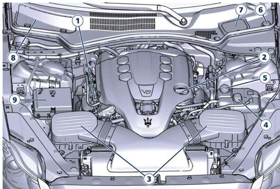
V6 – Moteur
