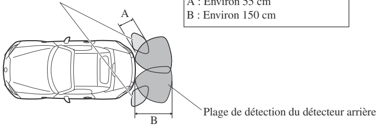
Plage de détection du détecteur de coin arrière
