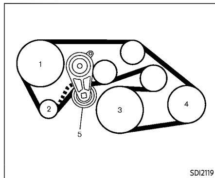
Moteur VQ37VHR
