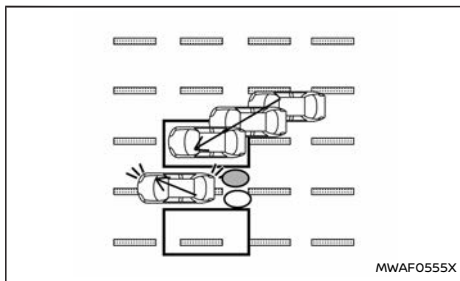
Illustration 6 – Entrée latérale dans le périmètre de détection
