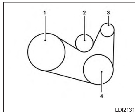
Moteur VQ35DD
