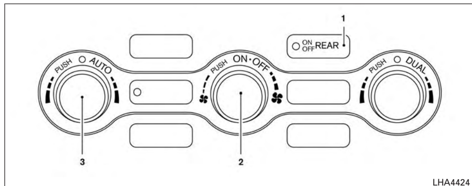
Commandes avant (type B, selon l'équipement)
