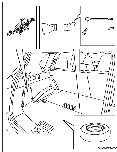
Modèle avec plancher de coffre réglable
