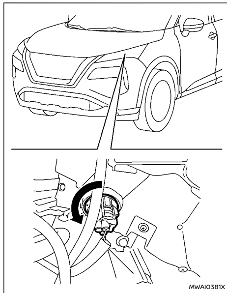
Clignotant avant (type à ampoule)
