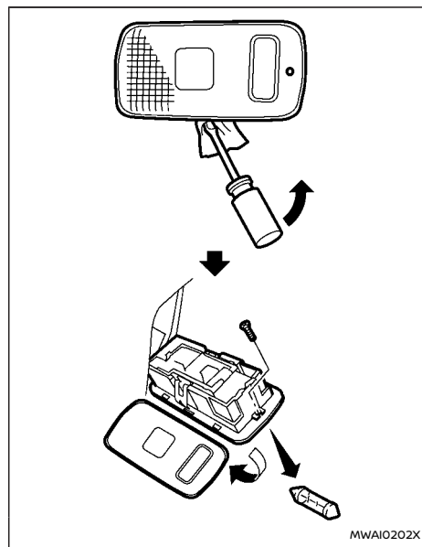
Éclairage de coffre
