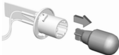
Feu stop (1)
