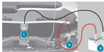
A. Point métallique positif de votre véhicule B. Batterie de secours
