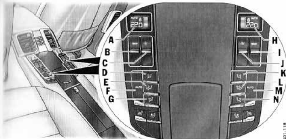
Panneau de commande arrière (climatisation 4 zones)
