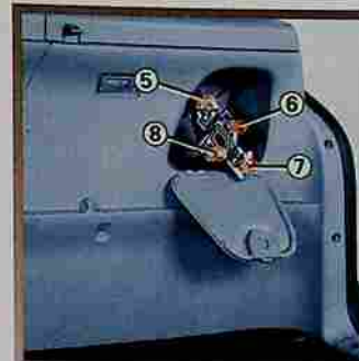
5 Feu de position et de stop Lampe forme poire à ergots P21/5W.
