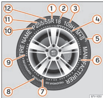
Fig. 303 Inscription universelle sur les pneus.
