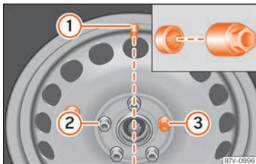
Fig. 70 Changement de roue : valve du pneu ① et emplacement du boulon antivol de la roue ② ou ③.
