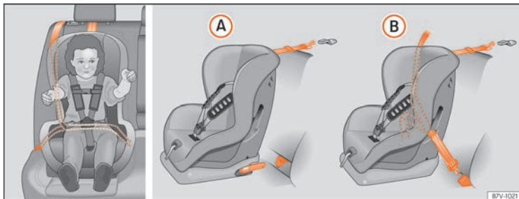
Fig. 38 Sur les sièges arrière : installations possibles d'un siège pour enfants.
