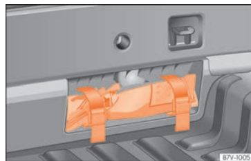
Fig. 101 Dans le coffre, vu depuis l'intérieur du véhicule : outillage de bord dans une cavité située dans la zone du porte-serrure.
