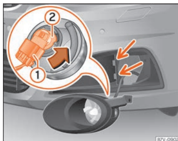
Fig. 112 Remplacement des ampoules des projecteurs.
