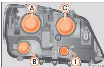
Fig. 107 Dans le compartiment moteur : revêtements dans le phare gauche. A feux de croisement, B feux de jour et C feux de route et feux de position.
