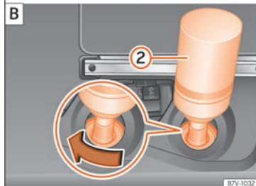
Fig. 289 Réservoir d'AdBlue avec bouchon de fermeture de la goulotte de remplissage et un bidon pour rajouter du liquide.
