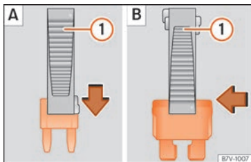
Fig. 64 Retirer ou placer un fusible.
