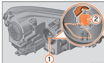
Fig. 110 Porte-ampoule du clignotant (1) et feu de virage (2).
