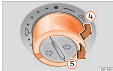
Fig. 16 Dans le ciel de pavillon : appuyer sur la commande et tirez-la pour lever et baisser le toit.
