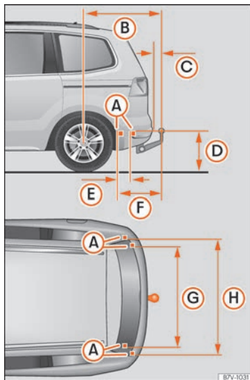
Fig. 282 Cotes et points de fixation pour l'installation ultérieure d'un dispositif d'attelage.
