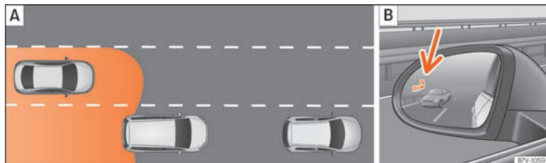
Fig. 273 Représentation schématique : A En cas de dépassement en présence de trafic à l'arrière du véhicule. B Indication de l'assistant d'angle mort sur le rétroviseur extérieur gauche.
