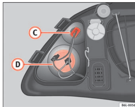
Fig. 141 Lampe du projecteur principal
