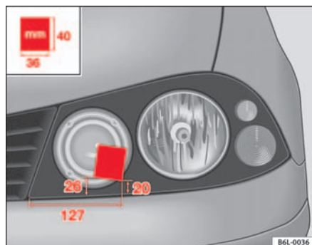
Fig. 114 Phare gauche
