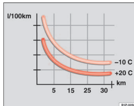
Fig. 117 Consommation de carburant (l/100 km) à deux températures ambiantes différentes. ►
