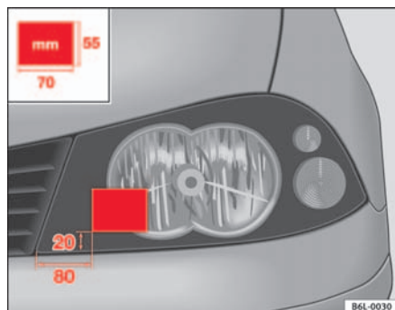
Fig. 108 Phare gauche
