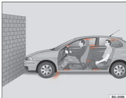
Fig. 6 Schéma de principe : véhicule se dirigeant droit sur un mur avec des occupants non sangles
