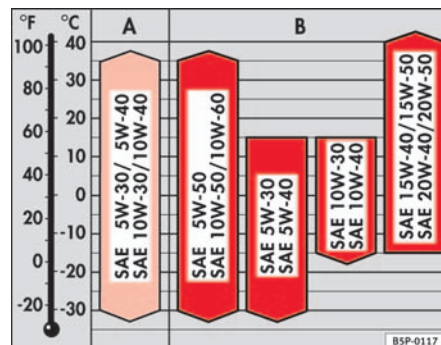
Fig. 121 Types d'huile en fonction de la température
