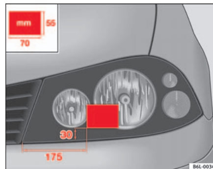
Fig. 112 Phare gauche
