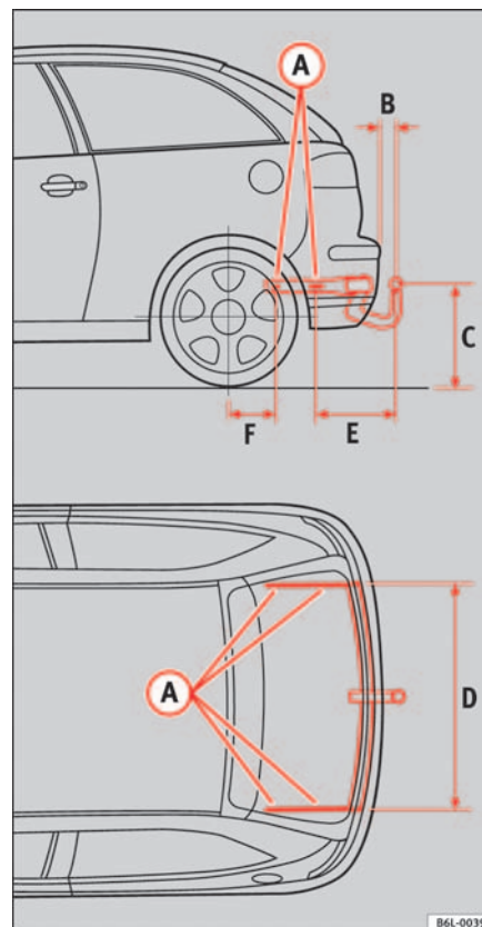
Fig. 118 Points de fixation du dispositif d'attelage
