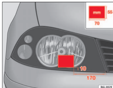
Fig. 107 Phare droit
