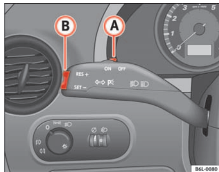
Fig. 103 Levier des clignotants et de l'inverseur-codes : commandes du régulateur de vitesse
