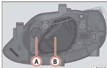
Fig. 187 Ampoules du phare AFS.
