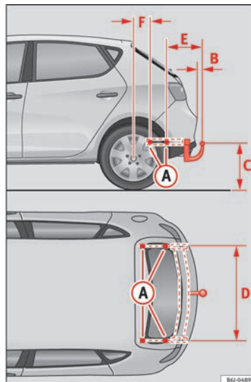
Fig. 150 IBIZA/IBIZA SC : points de fixation du dispositif de remorquage.
