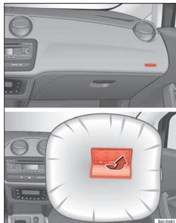
Fig. 57 Airbag du passager avant dans le tableau de bord.
