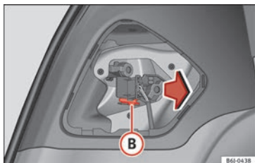
Fig. 199 Démontage du support d'ampoules.
