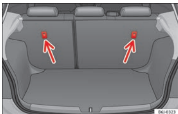
Fig. 67 Position des anneaux Top Tether sur la partie arrière de la banquette arrière.
