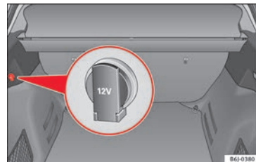
Fig. 115 Détail du revêtement latéral du coffre à bagages : prise de courant de 12 volts
