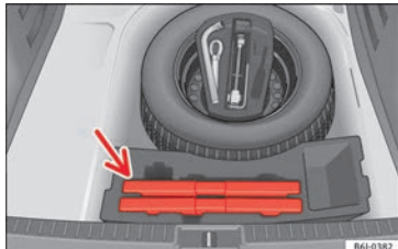
Fig. 156 Modèle IBIZA ST : logement pour le triangle de signalisation dans le coffre à bagages.
