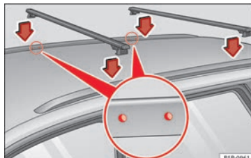
Fig. 124 Ibiza ST : points de fixation des barres longitudinales pour la galerie porte-bagages du toit.
