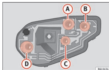
Fig. 194 Feu droit.
