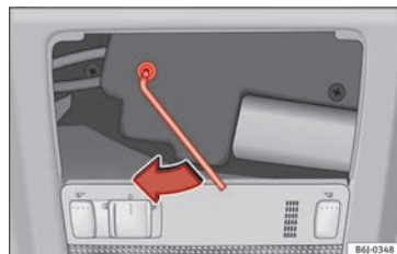
Fig. 88 Actionnement d'urgence du toit panoramique/relevable.
