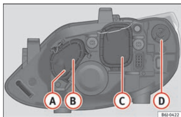
Fig. 179 Phare double.
