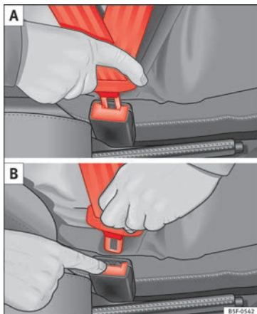
Fig. 54 Placer et retirer le pêne de verrouillage de la ceinture de sécurité.
