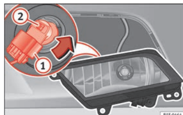
Fig. 192 Phare antibrouillard.
