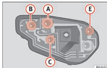
Fig. 193 Feu gauche.
