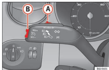
Fig. 149 Levier des clignotants et des feux de route : commande et touche basculante pour régulateur de vitesse.
