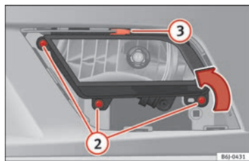
Fig. 190 Phare antibrouillard.
