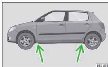
Fig. 134 Changement de roue : points d'appui du cric
