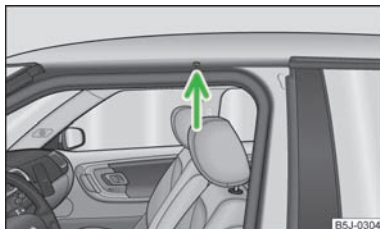
Fig. 58 Points de fixation des barres de toit de base
