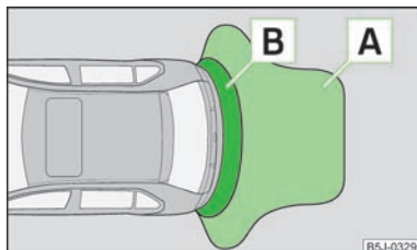
Fig. 83 Système d'assistance au stationnement : Portée des capteurs
