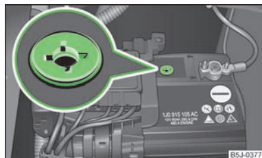
Fig. 124 Batterie du véhicule : indicateur de niveau de l'électrolyte
