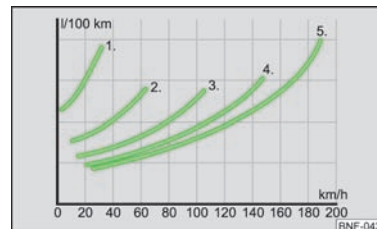
Fig. 111 Consommation de carburant en l/100 km en fonction du rapport engagé
