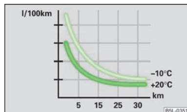
Fig. 113 Consommation de carburant en l/100 km à diverses températures
