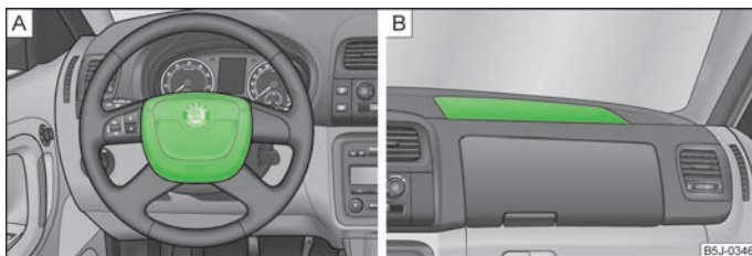
Fig. 100 Airbag avant du conducteur dans le volant/airbag avant du passager avant dans le tableau de bord
