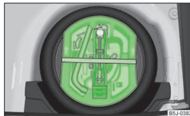
Fig. 132 Coffre à bagages : compartiment pour l'outillage de bord
