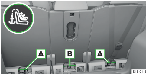
Œillets de fixation sur la banquette arrière VarioFlex
