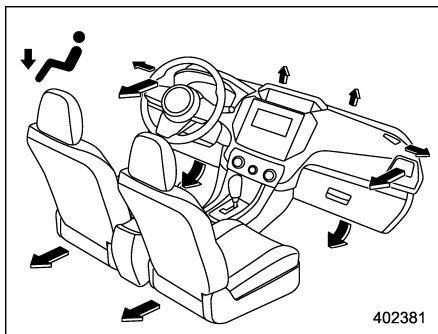
Chauffage: Sorties vers les pieds, sorties des deux côtés du tableau de bord et légèrement par les sorties du dégivreur du pare-brise (Une faible quantité d'air circule vers le pare-brise et les vitres des deux côtés pour éviter l'embuement.)
