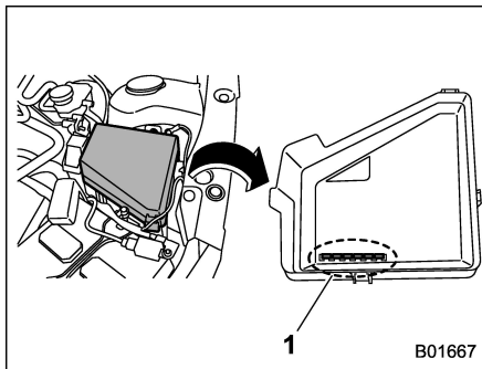
1) Fusibles de recharge
