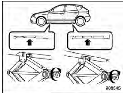
Points de levage (STI)
