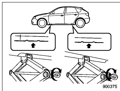
Points de levage (autres modèles)
