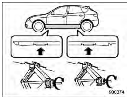
Points de levage (modèles équipés de bandeaux de marche, sauf STI)
