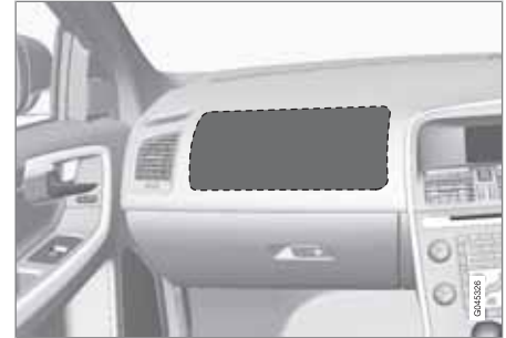
Emplacement du coussin gonflable du côté passager dans les voitures à conduite à droite.
