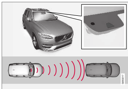
Emplacement de l'unité de radar et de la caméra.
